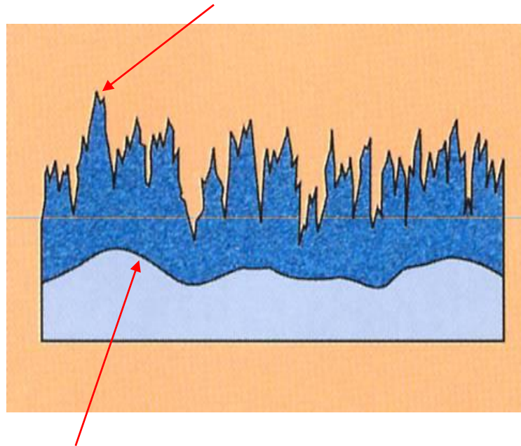
Nach Elektropolierung Abtrag ca. 20 \mu\text{m}
